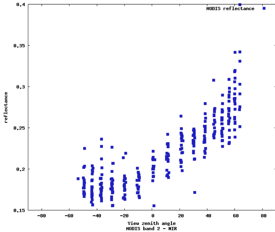
Band 2 (NIR)
