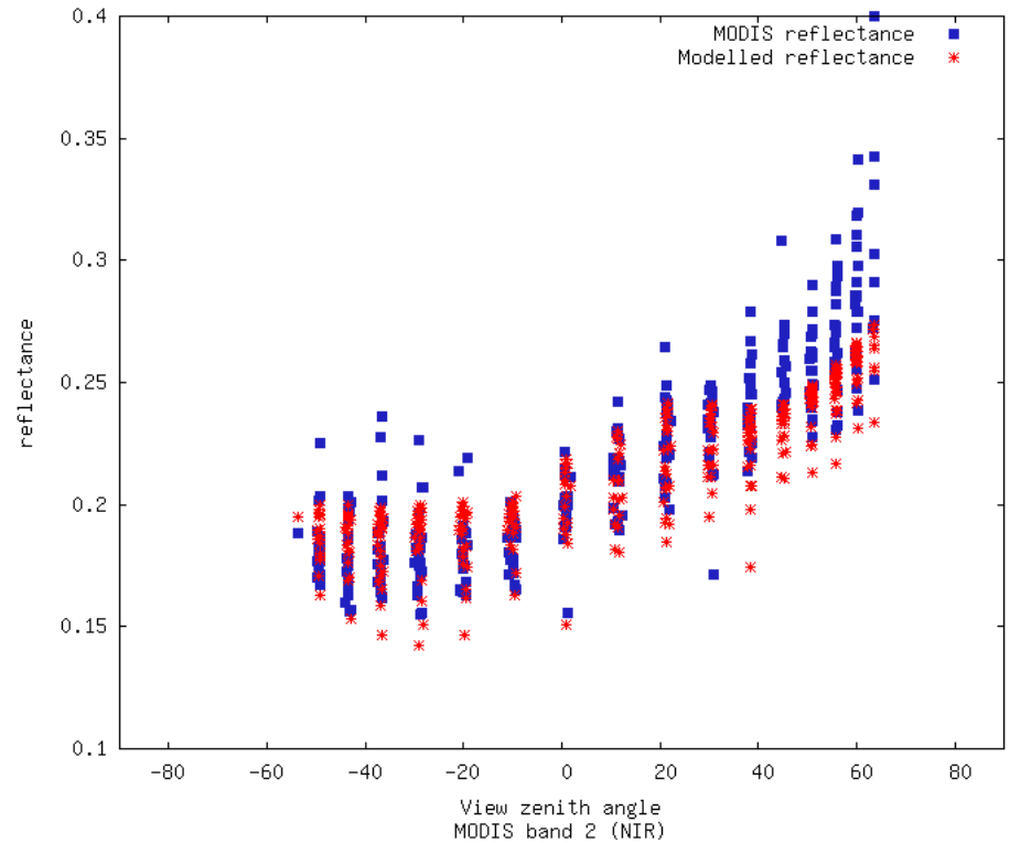
Band 2 (NIR)
