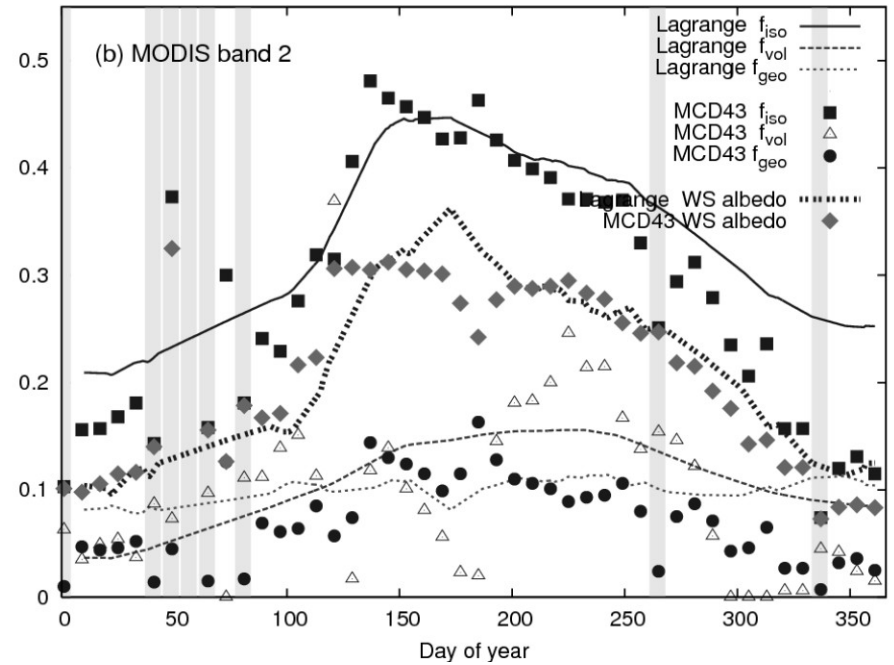
Band 2 (NIR)
